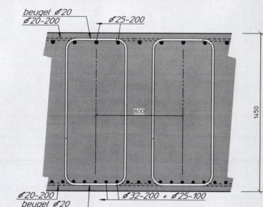
Doorsnede K-K
