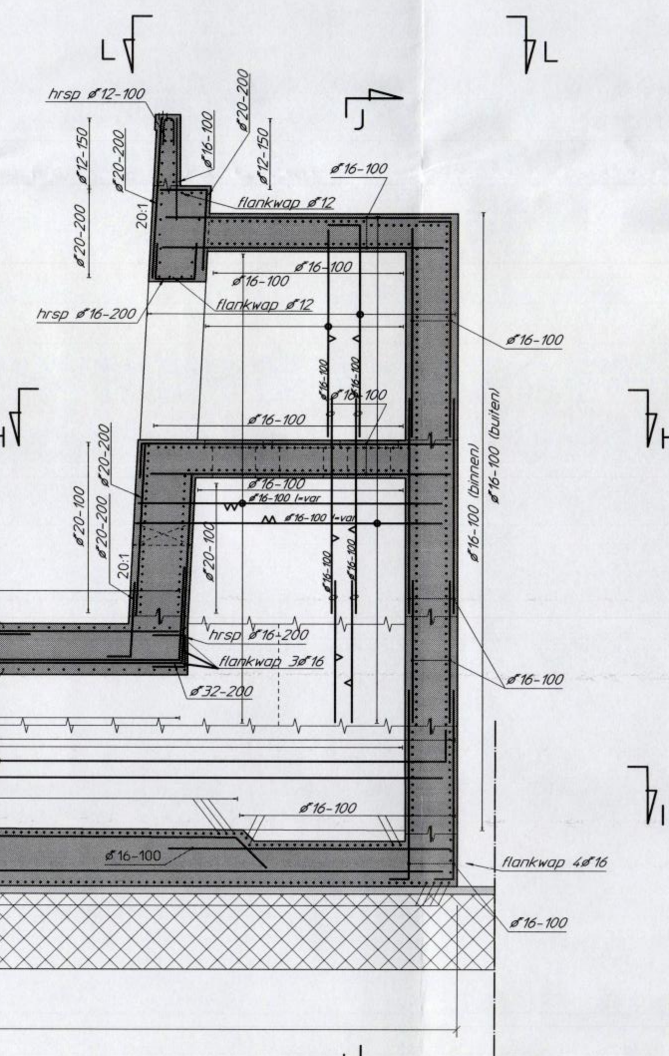
Aanzicht L-L
