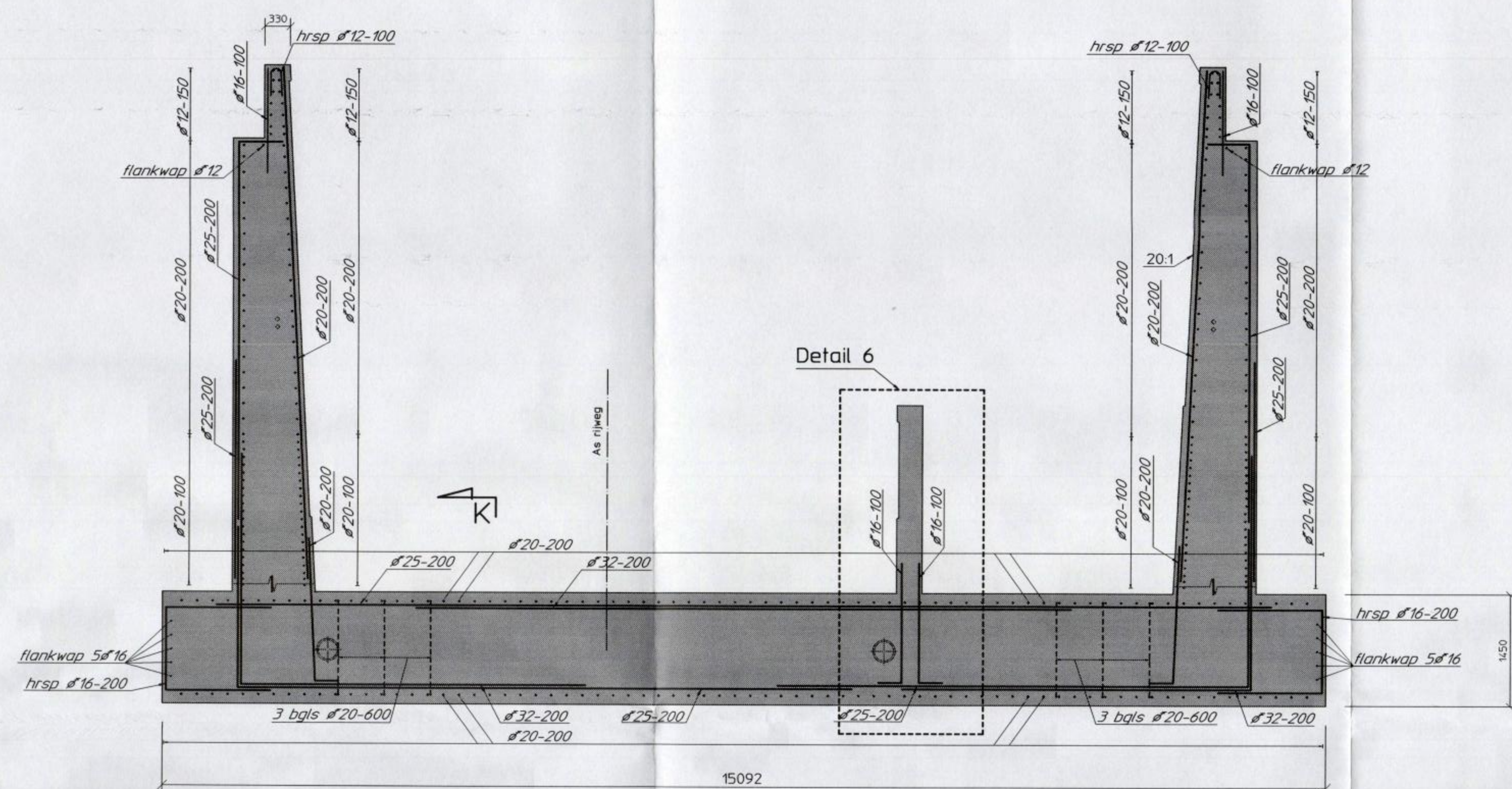
Doorsnede F-F
