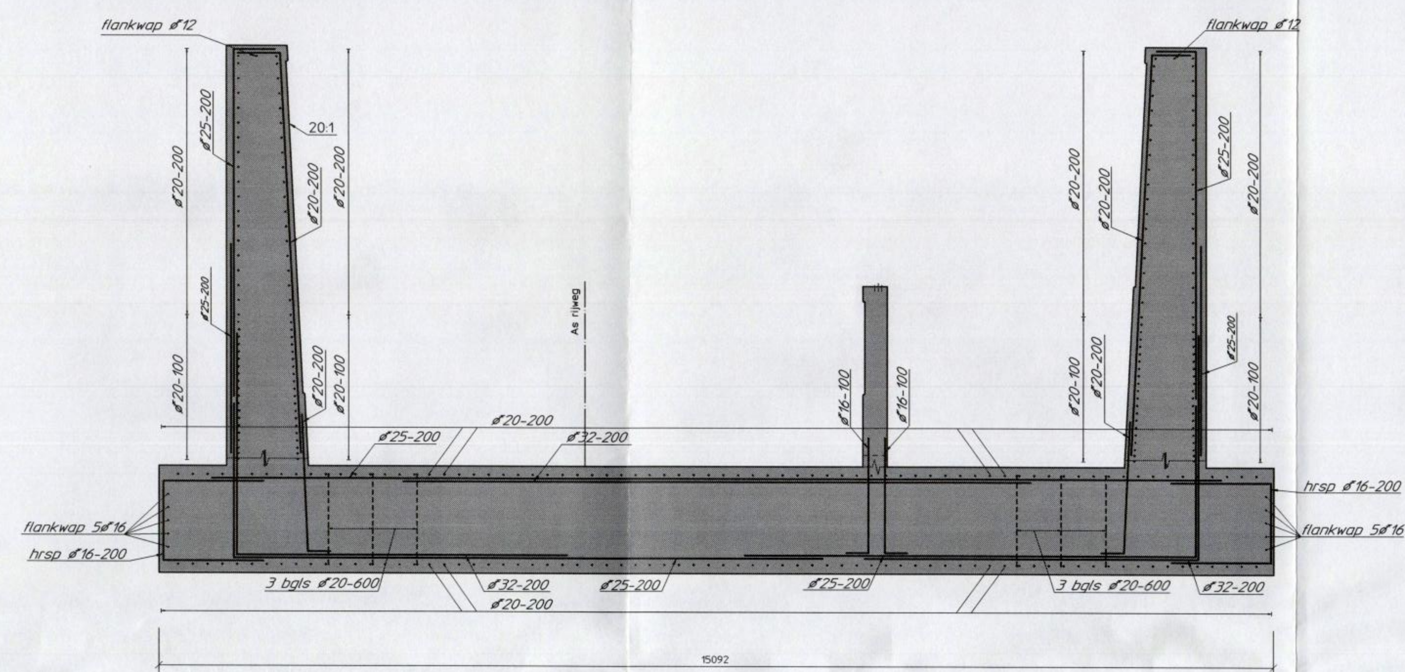
Doorsnede E-E
