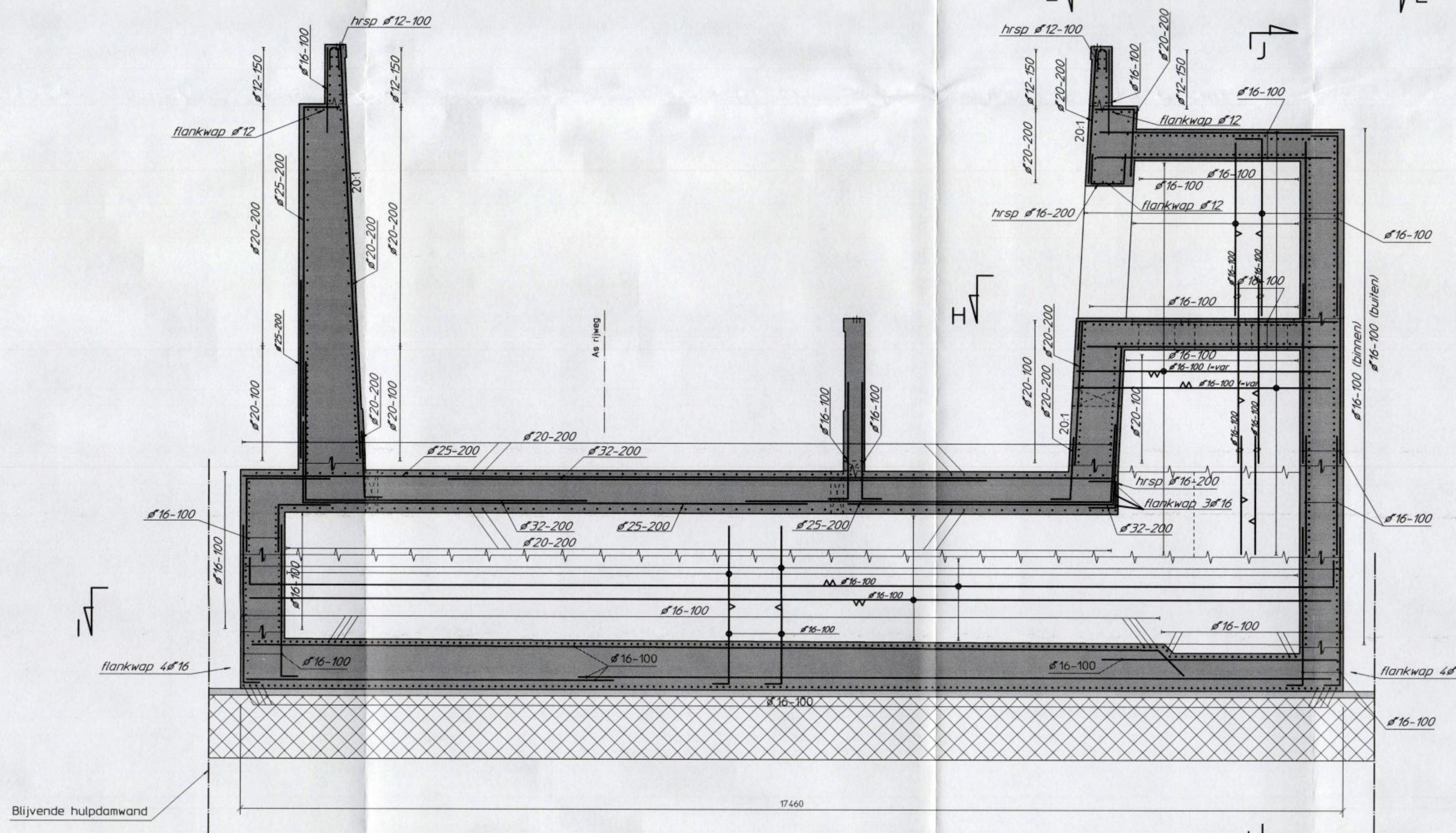
Doorsnede G-G
