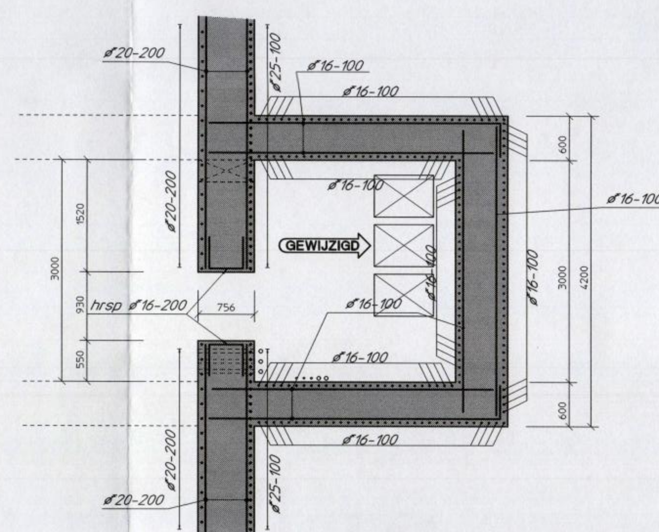
Doorsnede H-H
