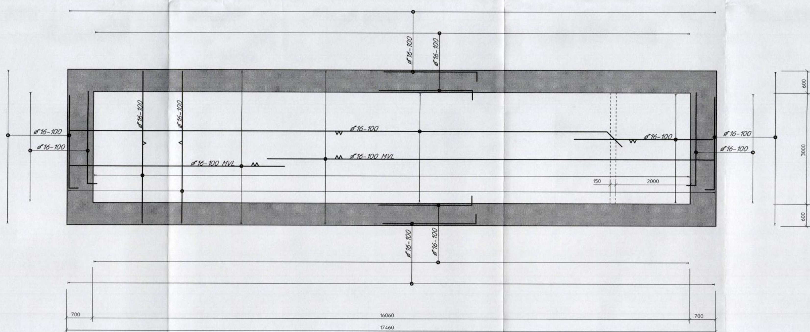
Doorsnede I-I
